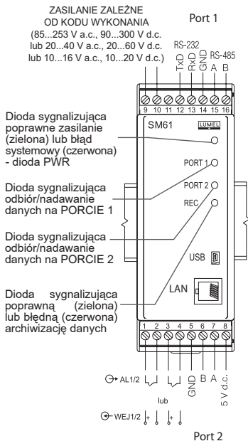
Rys. 3. Podłączenia elektryczne koncentratora SM61
