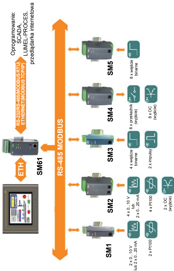
Rys. 1. Przykładowe zastosowanie koncentratora SM61
